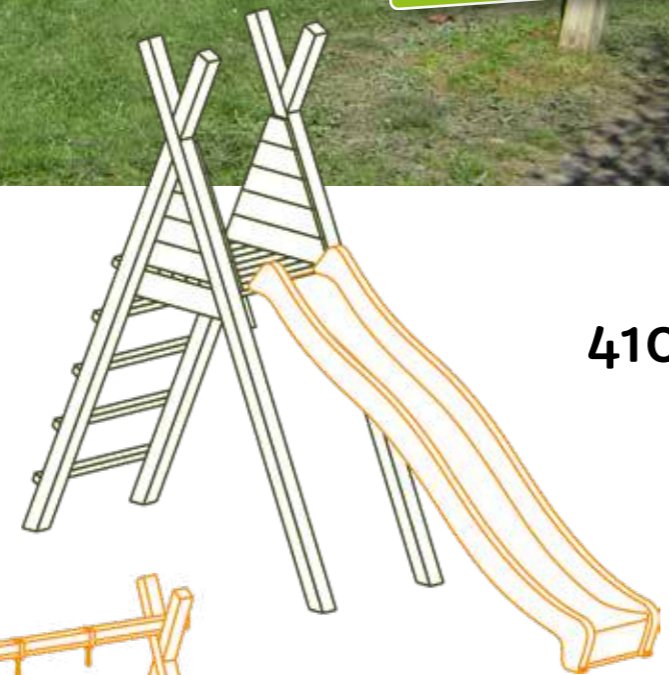
Afmetingen speeltoren: 5000 x 4150 mm
